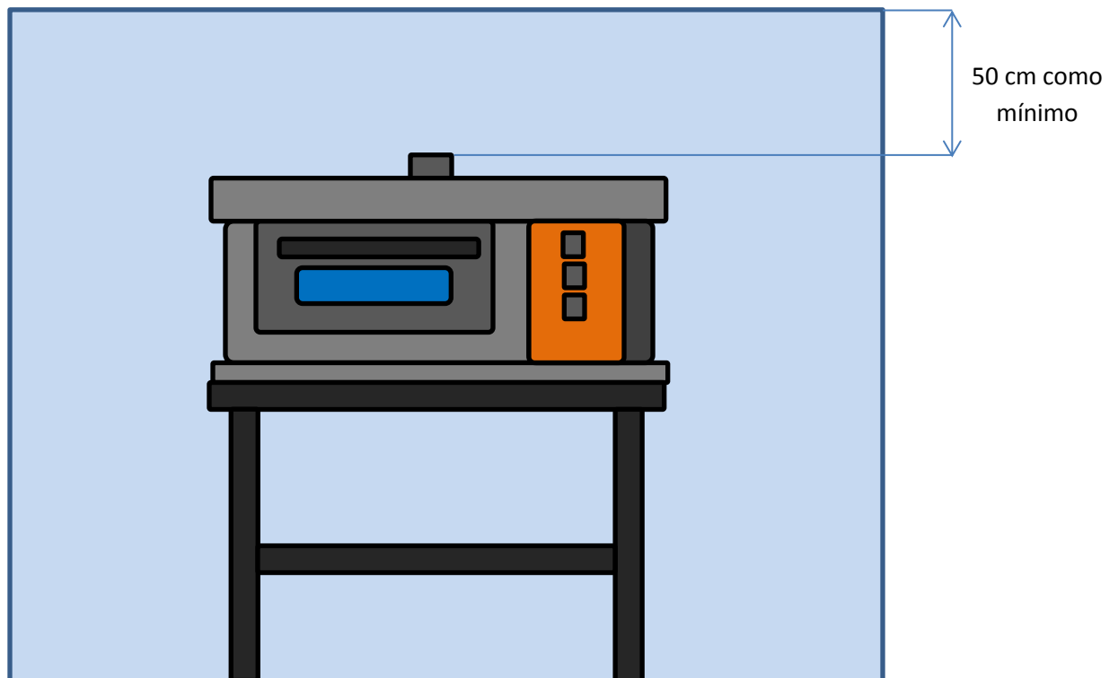
FIGURA 2. VISTA ALZADA HORNO
